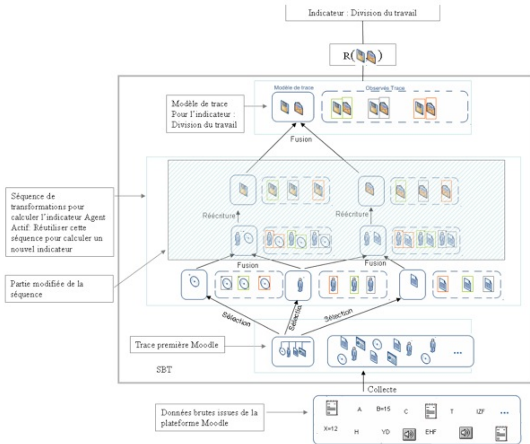
Figure 15 • Calcul d'un nouvel indicateur « division du travail » dans le SBT à partir d'une séquence qui existe dans la bibliothèque de modèles, issue de l'indicateur « Agent actif » par rapport à la trace première Moodle.
